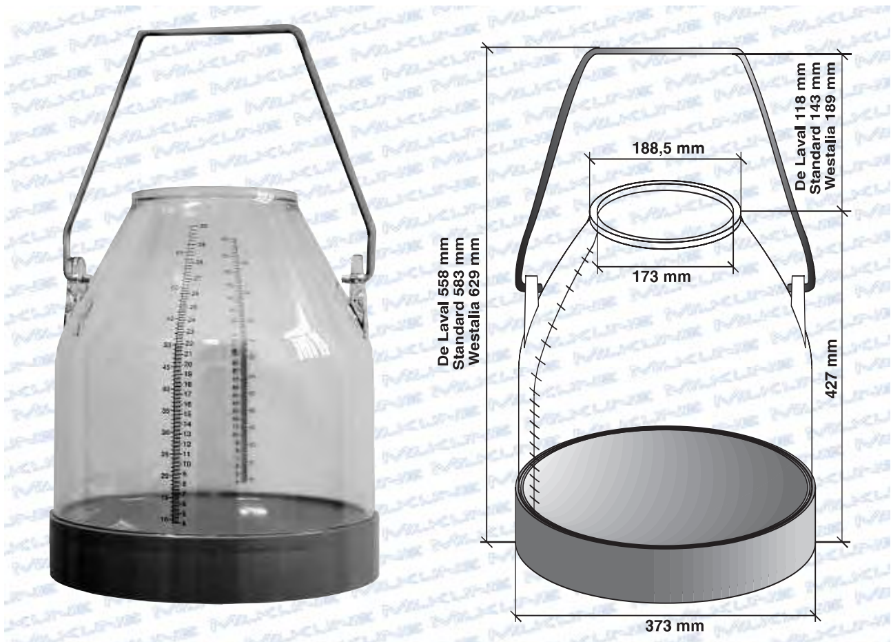
Secchi mungitori Milkline P30 con scala graduata Milkline P30 graduation milking buckets Milkline P30 Melkeimer mit Meß-Skala Pots trayeurs Milkline P30 avec graduation
